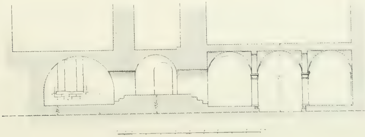
Fig. 52. Przekrój poprzeczny części podziem.
